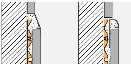
Variantes de instalación: Perfiles para delimitar el área calefactada de pared Schlüter®-DESIGNLINE Schlüter®-RONDEC
